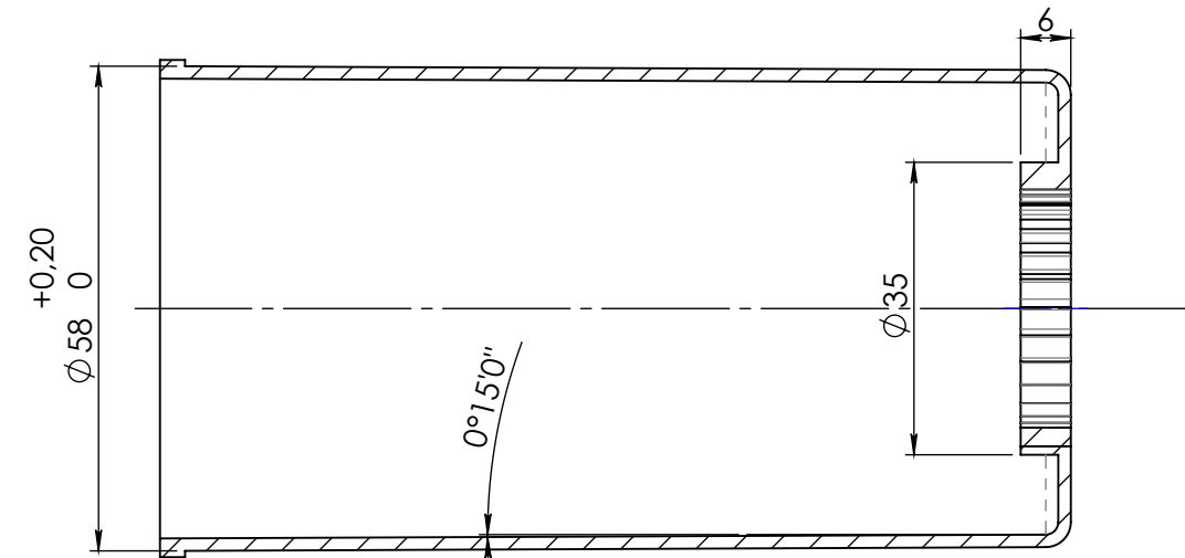
A-A
